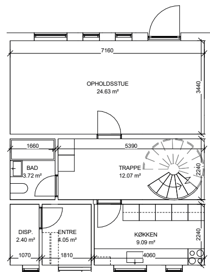
Stueplan
