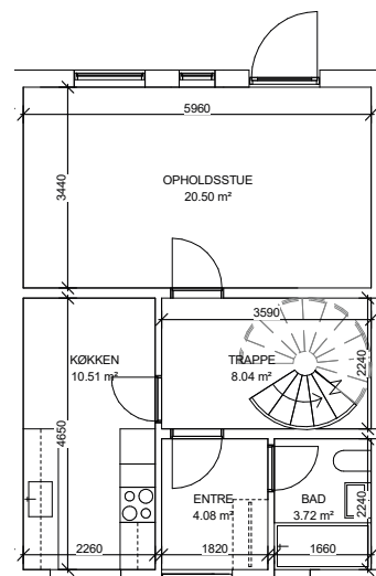
Stueplan
